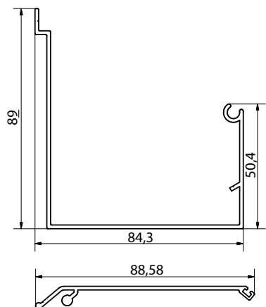
PROFILO GRONDA
