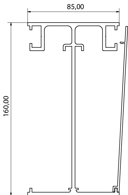
PROFILO GUIDA
