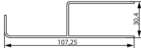
PROFILO COMPENSATORE
