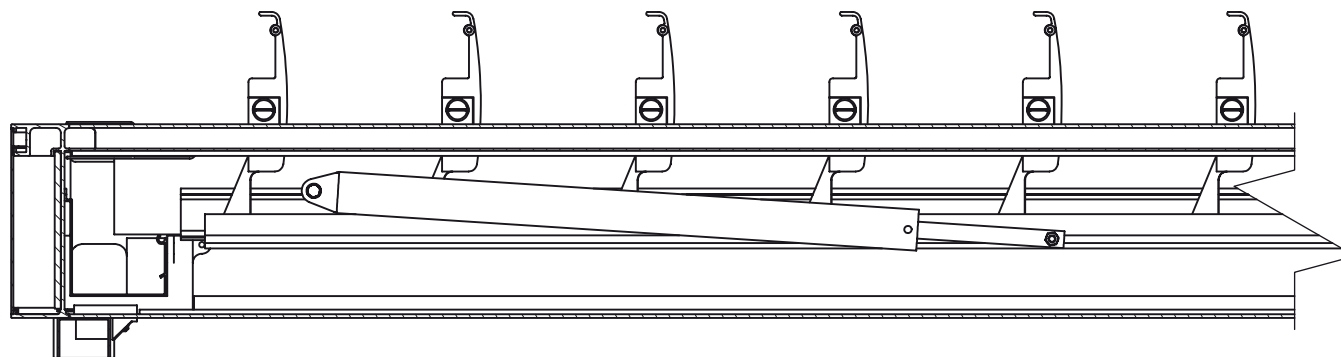
Manovra motore
